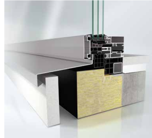
FWS 60 CV Baukörperanschluss
